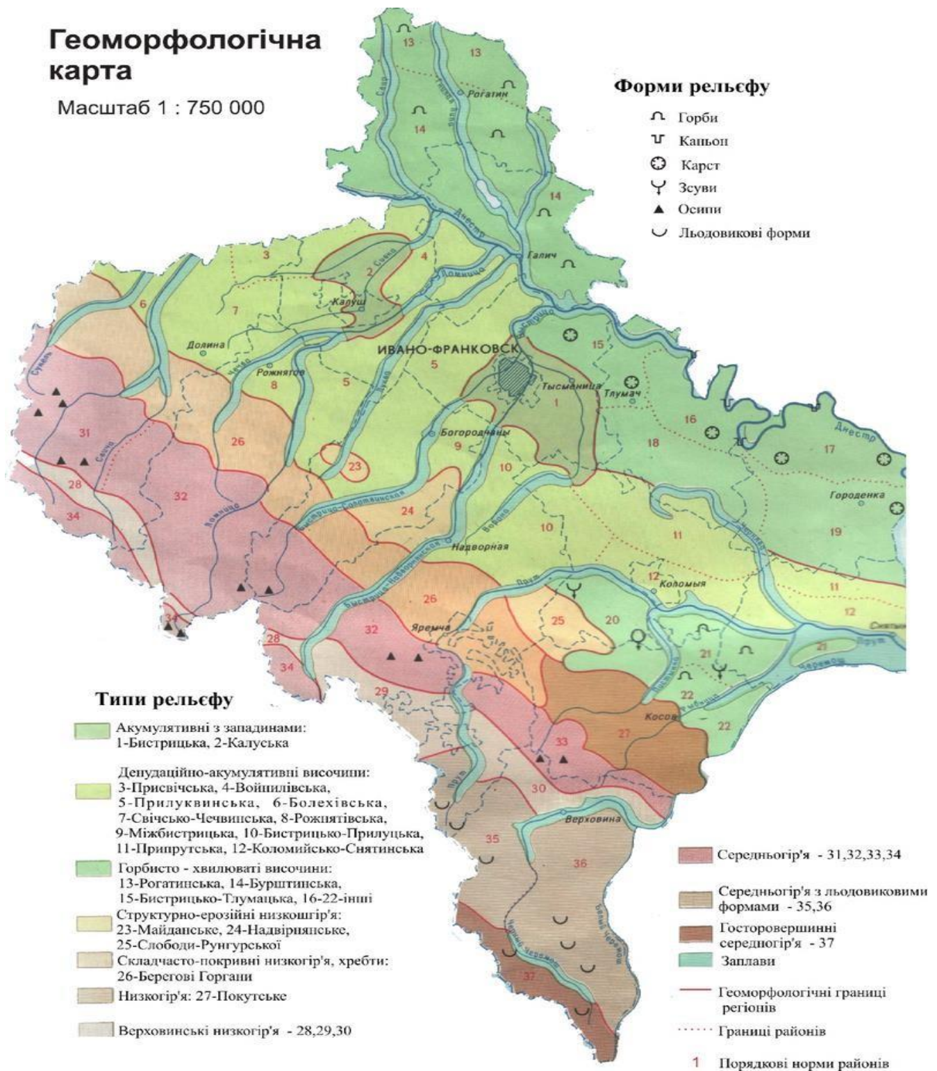
Рис. 1.2.1. Фрагмент фізичної (геоморфологічної) карти з відображенням території Івано-Франківської області
