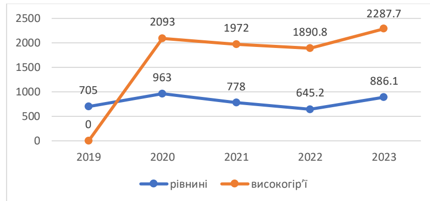
Рис. 1.2.3. Динаміка річної кількості опадів по області з 2019-2023 роки. https://www.if.gov.ua/dovkilliya
