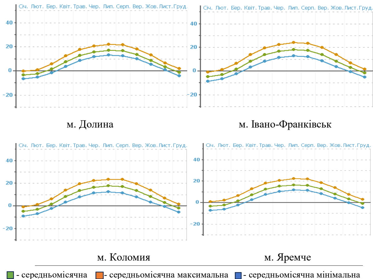
Рис. 1.2.4. Середня місячна і річна температура повітря деяких міст Івано-Франківської області (°C)
