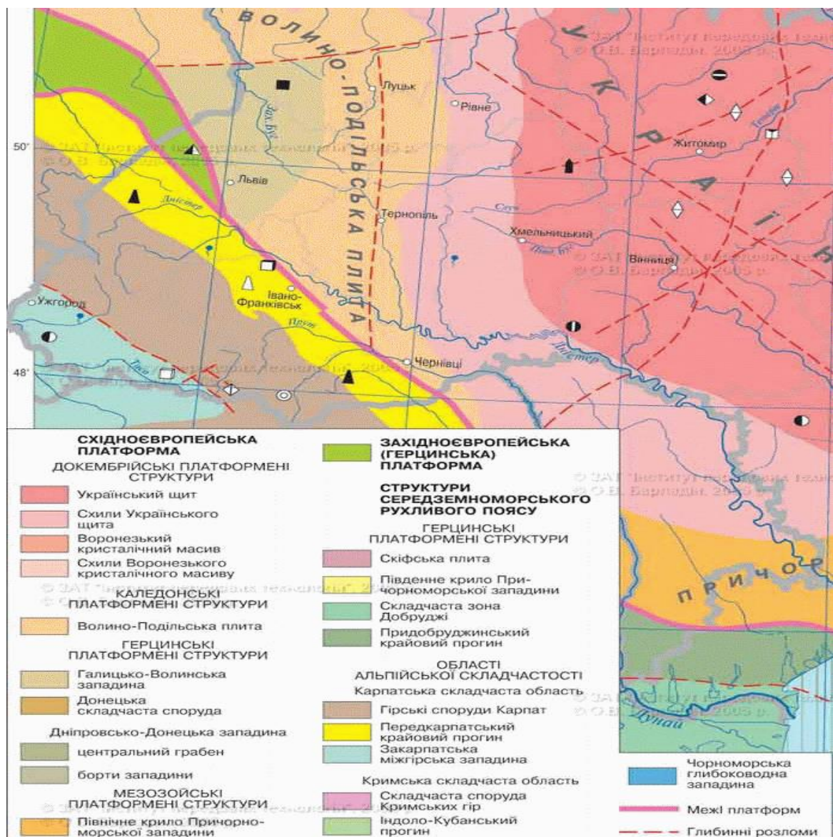
Рис. 1.2.2. Фрагмент карти тектонічної будови України з відображенням території Івано-Франківської області
