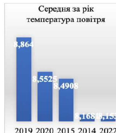
Рис. 2.3. Середня за рік температура повітря та її аномалія відносно кліматичної норми 1991–2020 років (а) та рейтинг 5-и найтепліших років із 1961 року (б) в Івано-Франківській області
