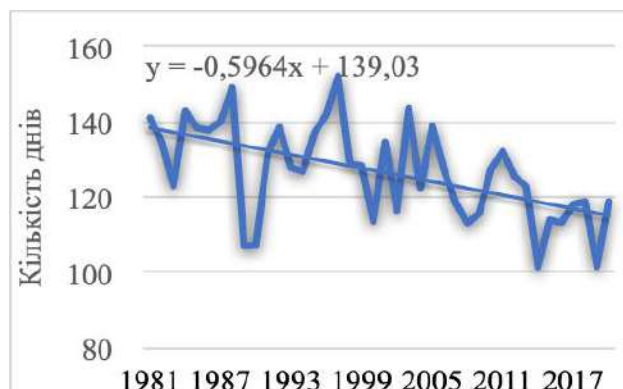
а) кількість морозних днів ( T_{\text{ср}} < 0^{\circ}\text{C} )
