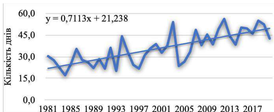
Рис.2.8. Кількість спекотних днів ( T_{\max} \geq 25^\circ\text{C} ) в Івано-Франківській області у період 1981-2020 з лінійним трендом
