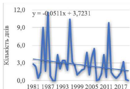
Рис. 2.6. Динаміка кількості днів з екстремальними температурними умовами у холодний період в Івано-Франківській області у період 1981-2020.
