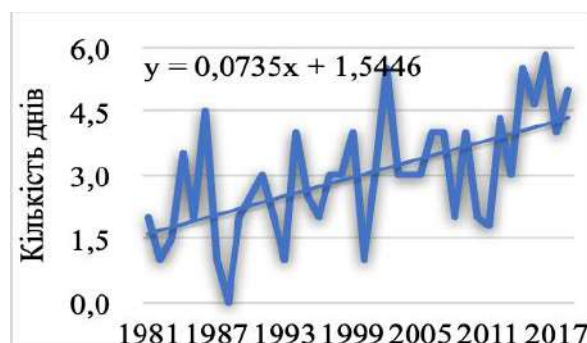
б) кількість днів з градом
