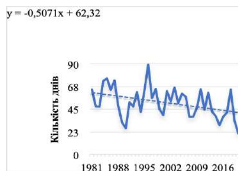
б) кількість днів з від'ємною максимальною за добу температурою ( T_{\text{макс}} < 0^{\circ}\text{C} )
