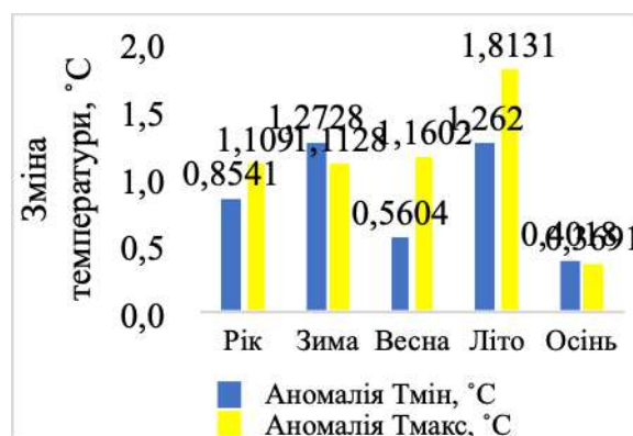
Рис. 2.5. Зміна (аномалія) середньої максимальної та мінімальної за рік, сезон та місяць температури повітря у 1991-2020, відносно 1961-1990 в Івано-Франківській області
